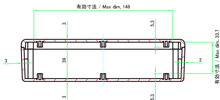
B-B ( 1 : 2.5 )
