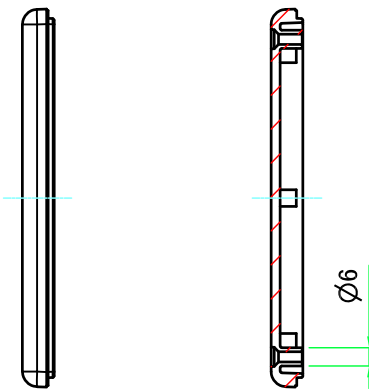
C-C ( 1 : 2.5 )
