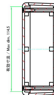
A-A ( 1 : 2.5 )
